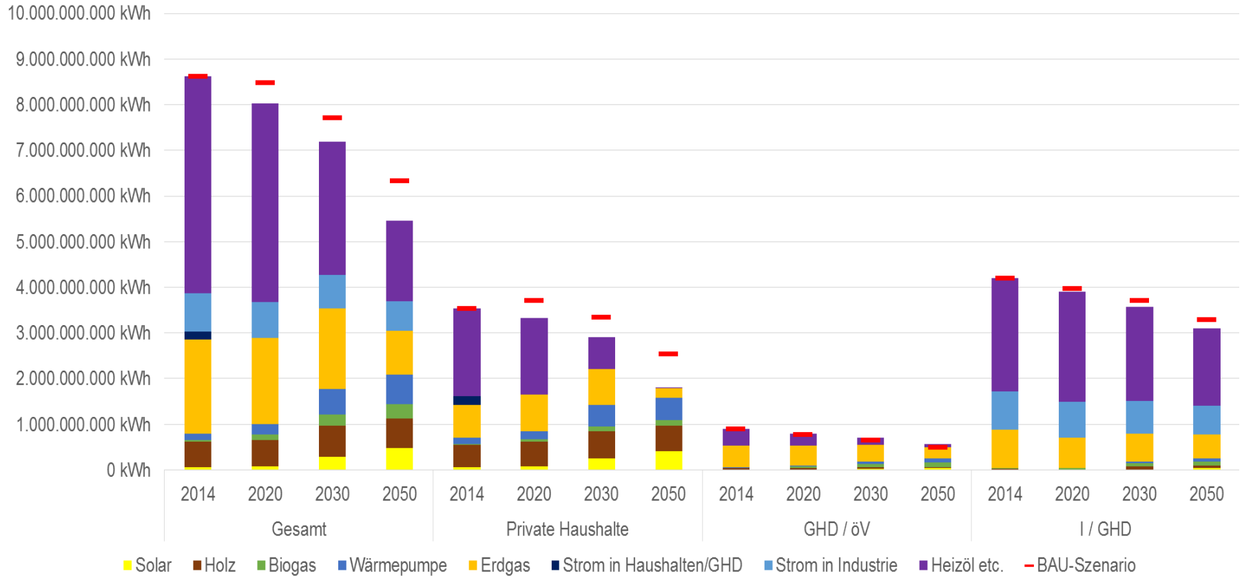
Entwicklung des Wärmebedarfs nach Energieträgern im regional basierten Szenario
