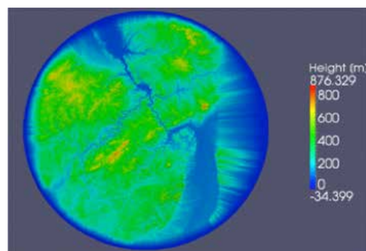
Abb. 7: Darstellung der Orographie im Modellgebiet
