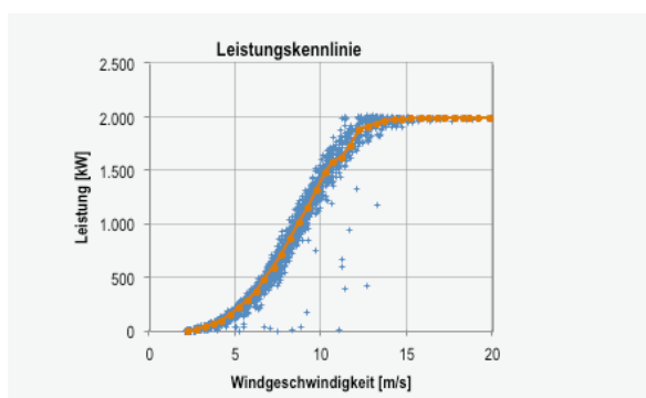
Abb. 11: Leistungskennlinie einer 2 MW Anlage
