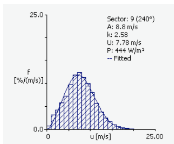
Abb. 10: Beispiel einer Weibullverteilung
