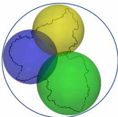
Abb. 6: Modell- und Kerngebiet der Berechnung.
