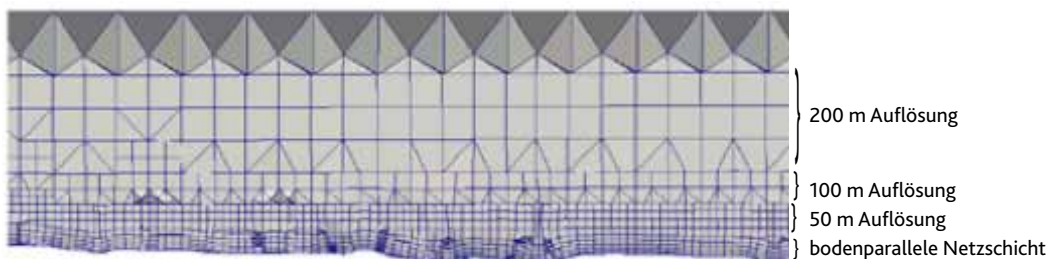
Abb. 5: Vertikaler Schnitt durch das Modellgitter.
